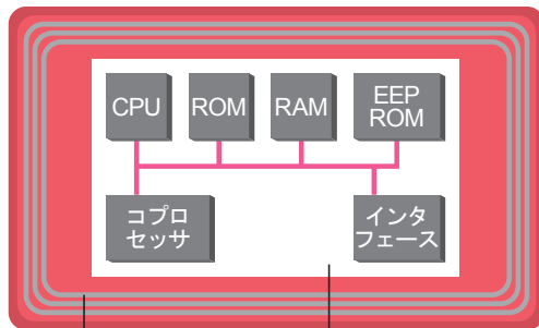
コイルアンテナ 半導体チップ (カード内に埋め込まれている)
